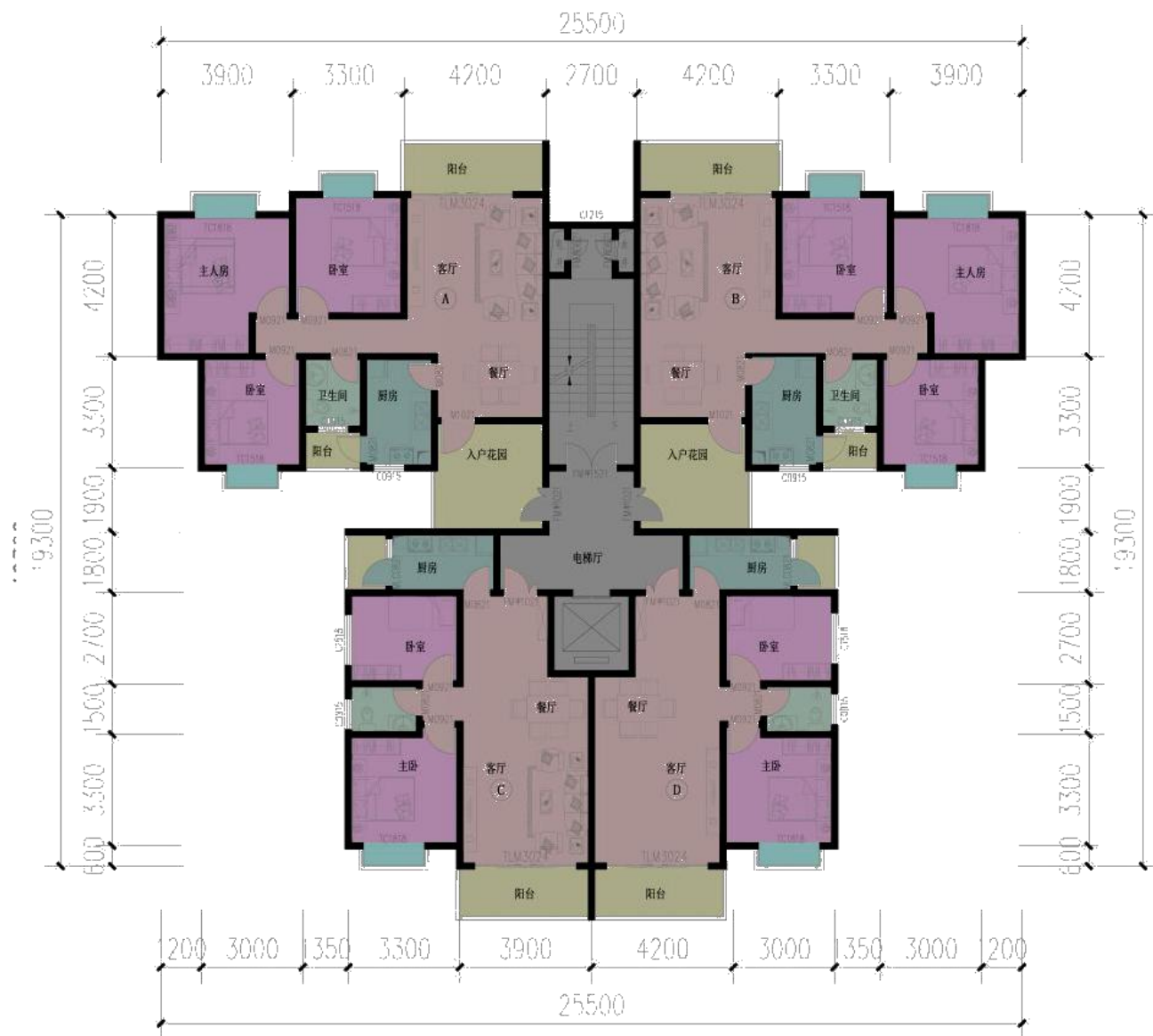
C#楼平面图 1:250
