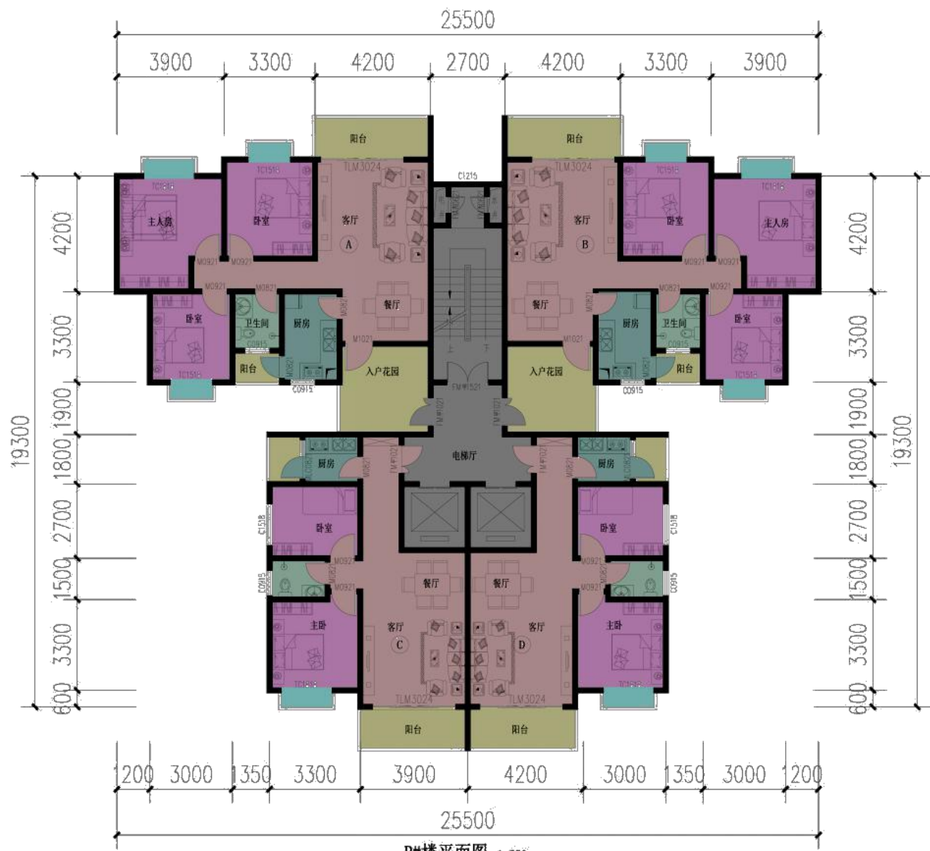
B#楼平面图 1:250
